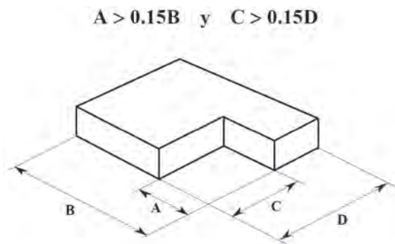
Figura 2. Irregularidad en planta por retrocesos en las esquinas.
