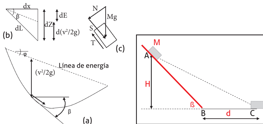
Figura 3-11. Bloque deslizante, consideraciones dinámicas. a) Perfil de la trayectoria. b) Geometría local del contacto. c) Diagrama de fuerzas. d) Planteamiento del problema.
